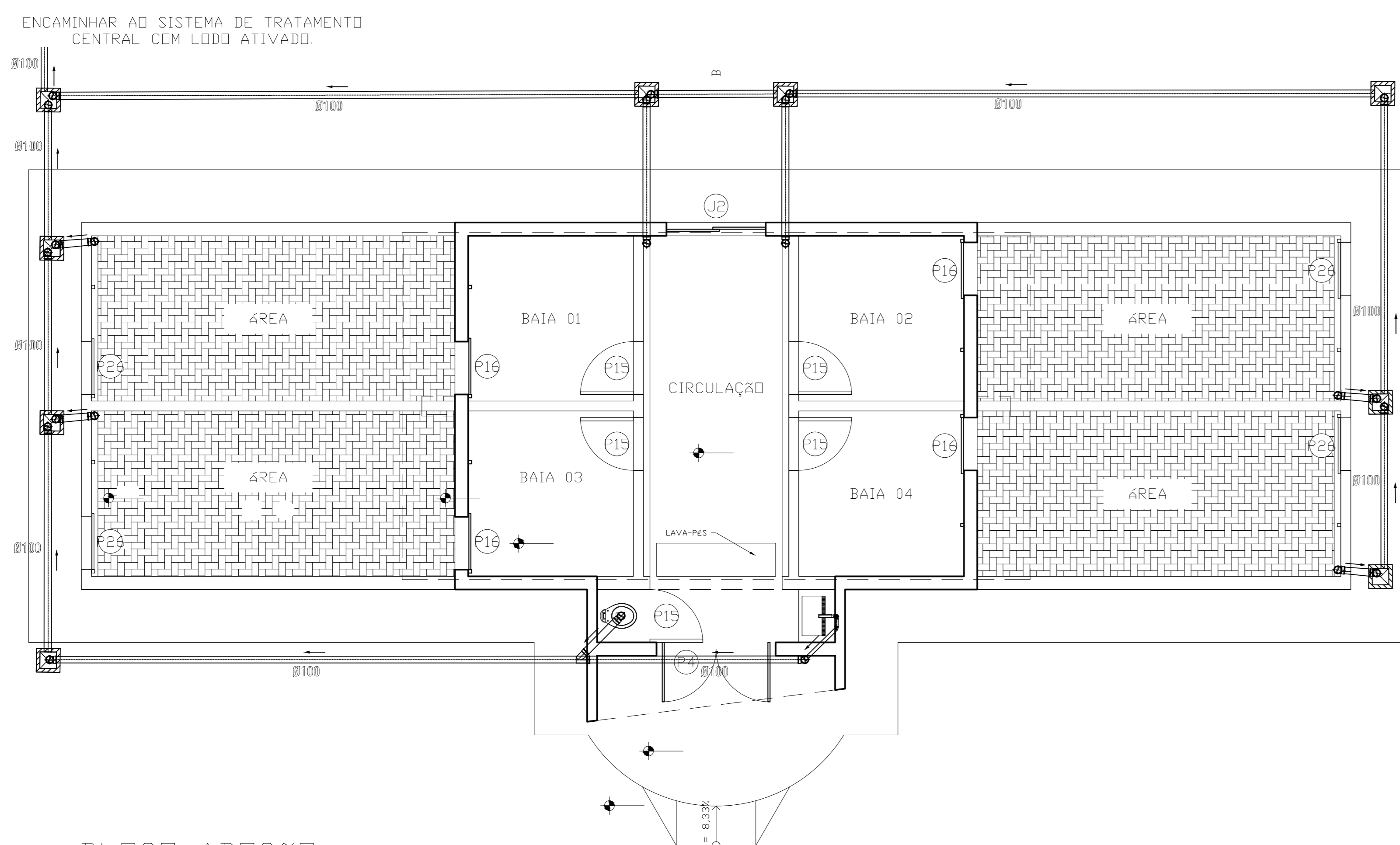
BLOCO ADOÇÃO ESGOTO SANITÁRIO ESCALA 1:50
