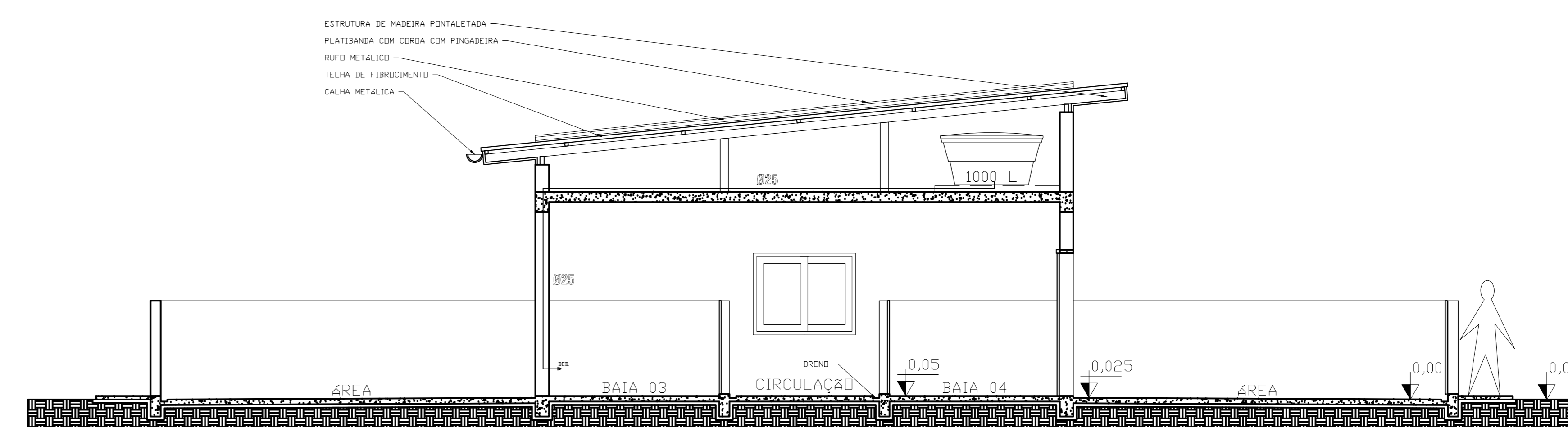
BLOCO ADOÇÃO ABASTECIMENTO ESCALA 1:50
